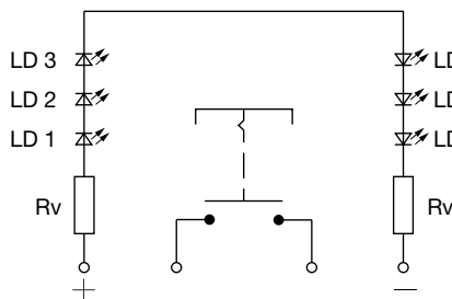
Kontaktbelegung zweipolig
