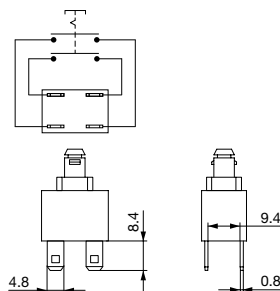
Kontaktbelegung zweipolig
